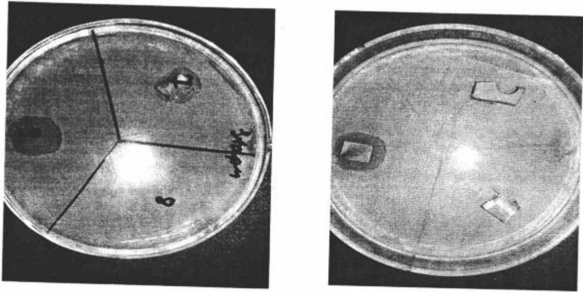
Фиг. 4 – Определение антимикробной активности титановых и стальных имплантатов методом диффузии
